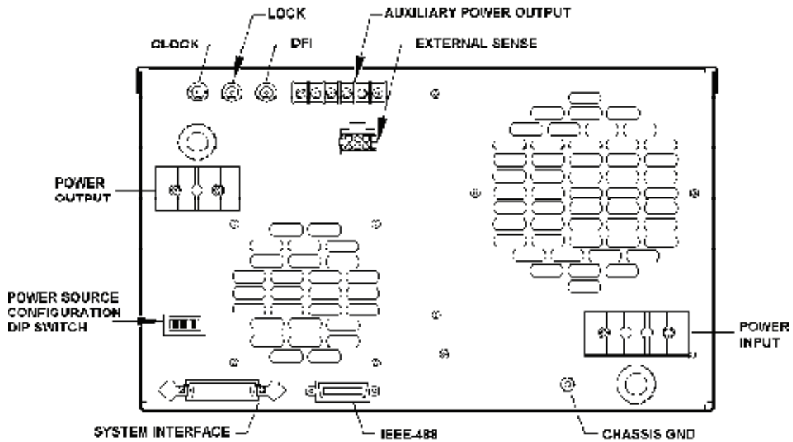
2750L / 4500L / 6000L REAR PANEL
